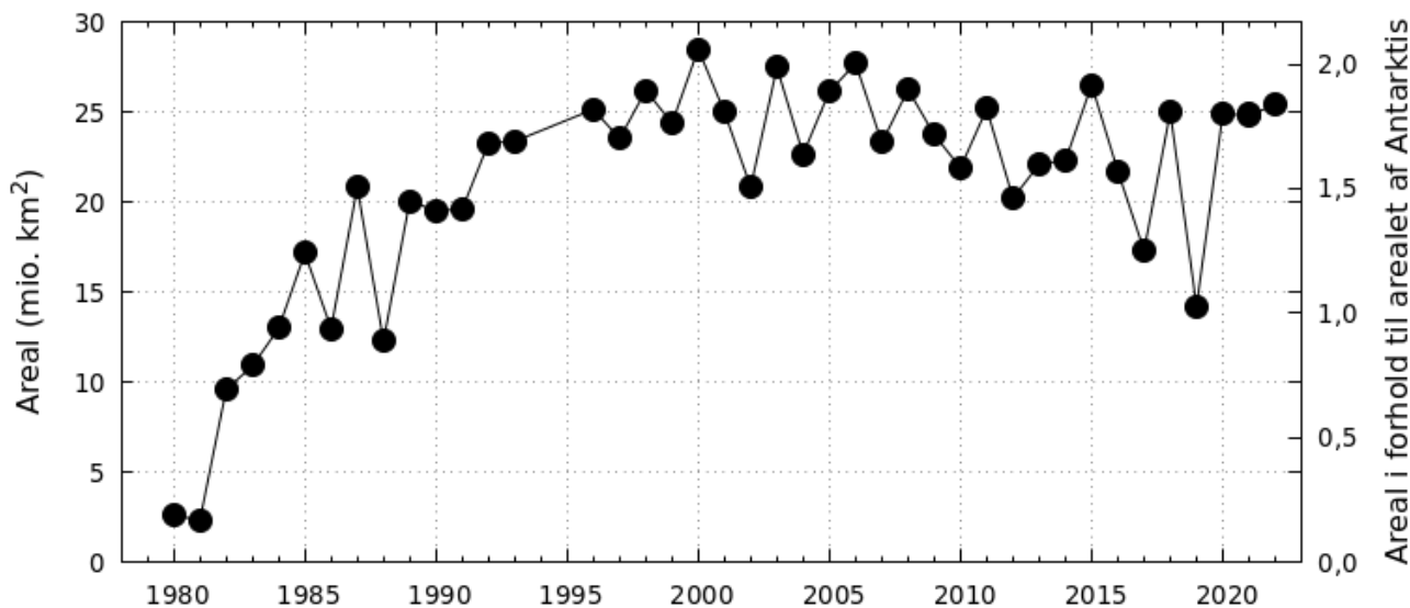
Fig. 4.3: Det maksimale areal af det antarktiske ozonhul i perioden 1979-2022.
