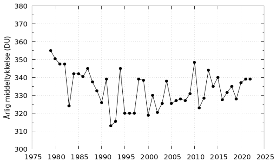
Fig. 1.3: Ozonlagets årlige middeltykkelse over Danmark for perioden 1979-2022. Den gennemsnitlige årlige middelværdi for 10-årsperioden 1979-1988 er 344 DU. Data fra før 1993 er data fra NASA's TOMS-instrument på Nimbus-7-satellitten. Data fra og med 1993 er DMI's målinger i København med et Brewer-spektrometer.
