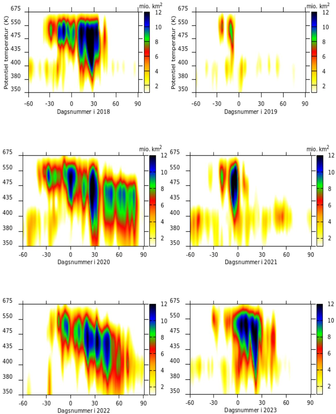
Fig. D5 – Areal af PSC'er i 2018-22. Som det ses af figuren, var der i vinteren 2018-19 ikke megen dannelse PSC'er. Arealet var maksimalt frem til slutningen af december. Herefter nedbrød en pludselig opvarmning ('sudden warming') den arktiske hvirvel, og et par uger efter slog et kuldefrembrud igennem på især USA's østkyst. Vinteren 2019-20 bød derimod på en meget lang periode med PSC'er - faktisk helt frem i april, hvor beregning af PSC-areal er ophørt, jfr. Appendix I. I vinteren 2020-21 var PSC området meget lille i hele perioden for mulig ozonnedbrydning. I 2021-2022 var PSC området det største siden 2005. Vinteren 2022-2023 havde et meget stort PSC område i januar, men det svandt hurtigt ind i februar.
