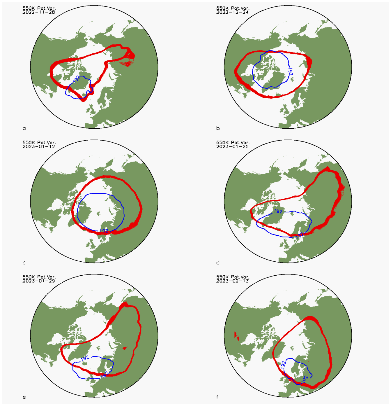
Fig. 2.1: Den polare hvirvel (røde konturer). Områder med type 1 PSC dannelse (tynde blå).
