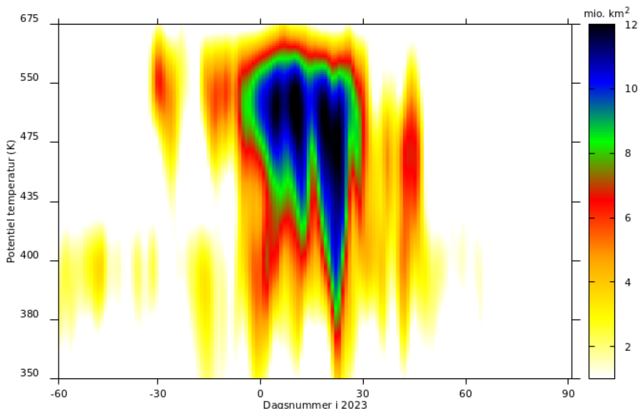
Fig. 2.3: Areal af den nordlige halvkugle dækket af PSC'ere i højdeinterval 350-675 K potentiel temperatur, svarende til ca. 14-26 km gennem vinteren 2022-2023. (ECMWF)
