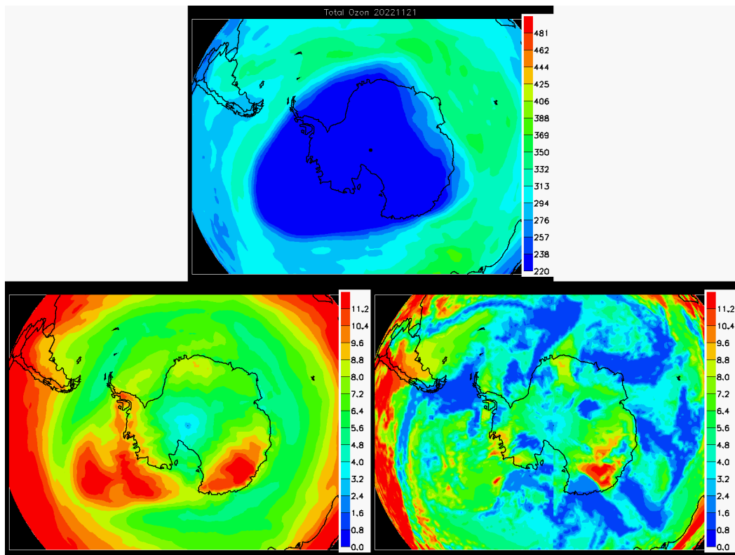
Fig. 4.6: Øverst: ozonhullets udbredelse 21/11 2022. Nederst tv.: UV indeks for skyfri himmel for samme dato. Th.: UV indekset korrigeret for skydække.
