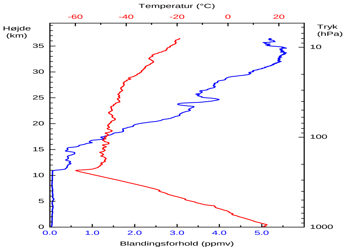
Figur F2. Ozon- og temperaturprofil fra Ittoqqortoormiit (Scoresbysund), Grønland, den 13. juli 1994 målt med en ozonsonde. Den samme profil som vist i figur F1, blot med en anden enhed for ozonkoncentrationen. Blandingsforholdet angiver, hvor mange ozonmolekyler der findes for hver million molekyler i den omgivende luft. Skala for ozon er nederst, for temperatur øverst.
