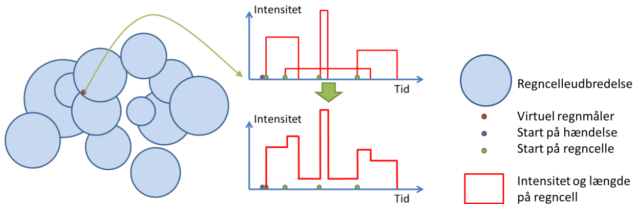
Figur 8.1: Skematisk repræsentation af den "spatio-temporale Neyman-Scott puls"-model. Venstre side repræsenterer et snap-shot af det spatiole modeldomæne på et givet tidspunkt og højre side viser den tidlige udvikling i et givet punkt i modeldomænet repræsenteret ved en virtuel regnmåler.
